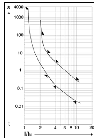
Für / For In 125 mA - 6,3 A ▽ Schmelzeit-Kleinstwert ▴ Schmelzeit-Größtwert
