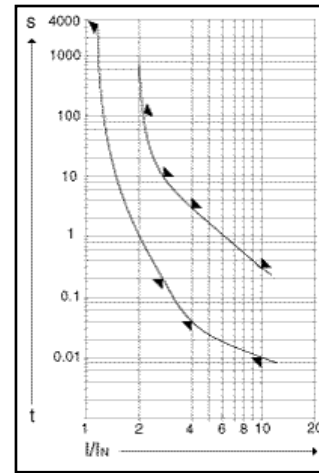
Für / For In 32 mA - 100 mA ▽ Schmelzeit-Kleinstwert ▴ Schmelzeit-Größtwert
