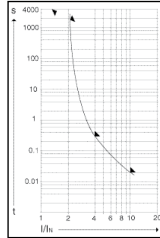
Für/For I_n 1,6 A - 6,3 A ▲ Schmelzeit-Kleinstwert ■ Schmelzeit-Größtwert
